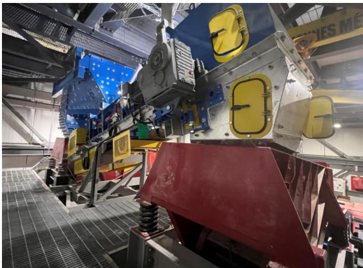
Goulottes, convoyeur et alimentateur du trieur de 3e minerai (gauche) ; installation de dépoussiérage (droite)
