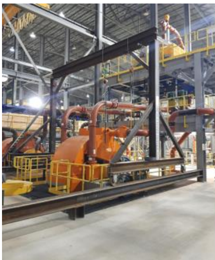
Nouveau WHIMS (à gauche) et espace de déchargement (à droite)
